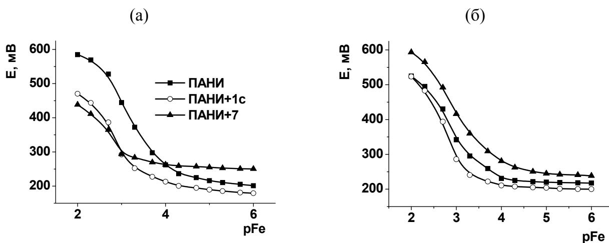
Рисунок 2. Зависимость потенциала ИСЭ на основе стеклоуглеродного электрода, покрытого ПАНИ и тиакаликс[4]аренами 1c и 7 , от концентрации ионов \text{Fe}^{3+} в яблочно-виноградном соке "Фруктовый сад" (а) и в яблочном соке "Rich" (б) при разбавлении 1:20 1 мМ сульфатом натрия.
