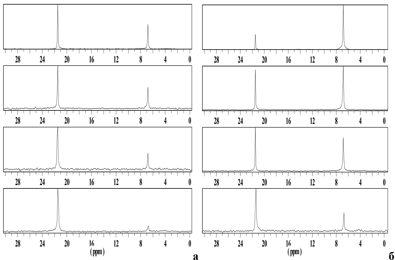
Рис. 7. Спектры ЯМР ^{31}\text{P} реакционных смесей p -хлорбензальдегида, анилина и диэтилфосфита через 5, 10, 15, 60 минут а) с изостевиолом, б) без изостевиола.
