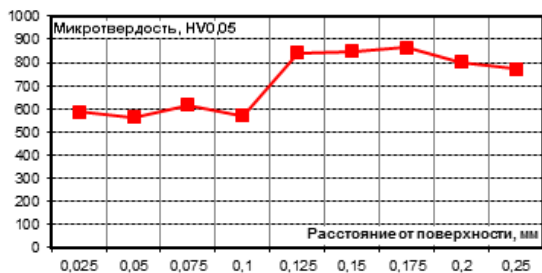
Рисунок 13. – График результатов замеров микротвердости в единицах HV 0,05 по глубине
