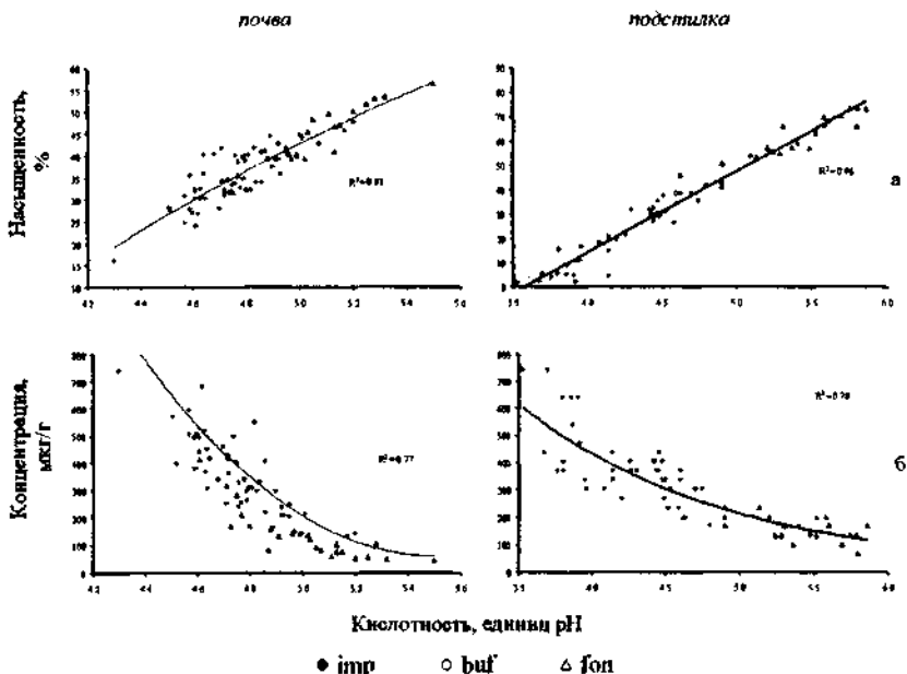
Рис. 17. Зависимость степени насыщенности основаниями (а) и содержания подвижного алюминия (б) от кислотности (рН водный) для образцов почвы и подстилки из фоновой (fon), буферной (buf) и импактной (imp) зон топоческой нагрузки. Субстраты отобраны по сетке 100х100 м (по 25 образцов в каждой зоне); учетная единица – образец.
