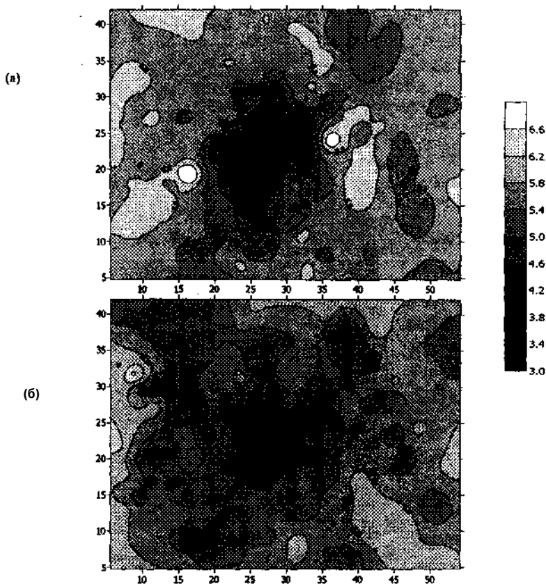
Рис. 3. Пример распределения фактической кислотности (единиц рН водный) лесной подстилки (а) и почвы (б) в районе действия точечного источника эмиссии загрязнителей (СУМЗ). По осям - расстояние в км.
