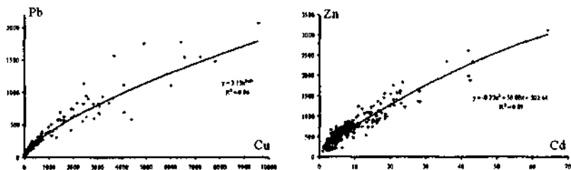
Рис. 6. Зависимость между концентрациями (мкг/г) подвижных форм (вытяжка 5%-ной HNO_3 отдельных элементов в лесной подстилке в масштабе всего градиента загрязнения (учетная единица - площадка). Район СУМЗа, отбор проб выполнен в 1995-1998 гг.
