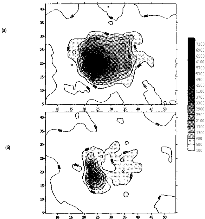
Рис. 2. Пример распределения содержания подвижных форм меди (мкг/г) в лесной подстилке (а) и почве (б) в районе действия точечного источника эмиссии поллютантов (СУМЗ). По осям - расстояние в км.
