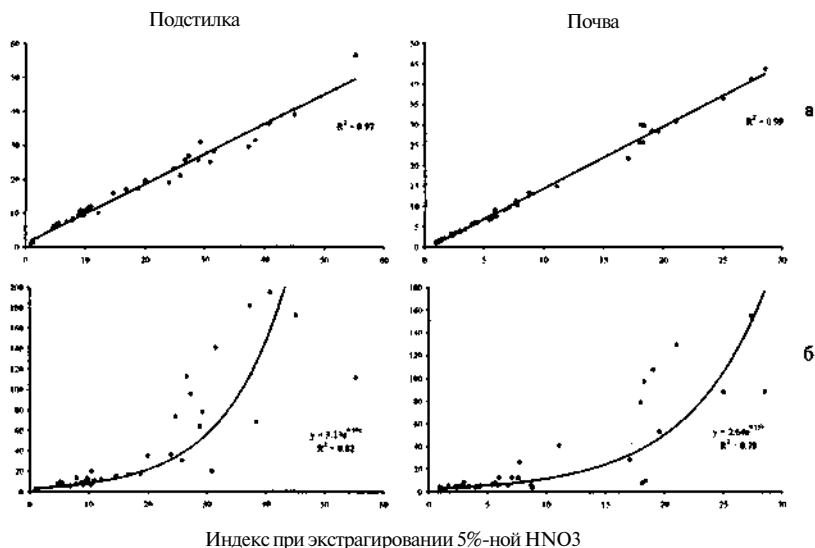
Рис. 8. Зависимость между индексами токсической нагрузки при использовании различных экстрагентов: а - раствор ЭДТА, б - раствор хлорида кальция. Учетная единица - площадка. Район СУМЗа, отбор проб выполнен в 1998 - 1999 гг.
