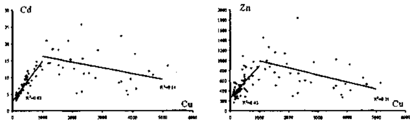
Рис. 7. Зависимость между концентрациями (мкг/г) подвижных форм (вытяжка 5%-ной HNO_3 отдельных элементов в лесной подстилке в масштабе всего градиента загрязнения (учетная единица - площадка). Район СУМЗа, отбор проб выполнен в 1990 г.
