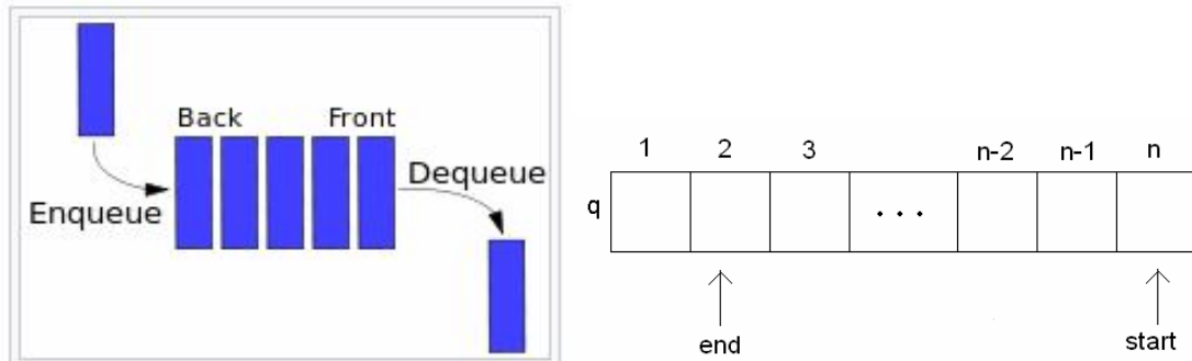
Рис. 4. Способы реализации очереди.
