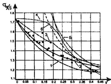
Рис. 3: Зависимость критической нагрузки от относительной толщины МП слоя, K = 1,74
