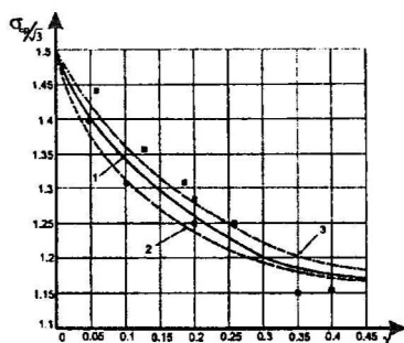
Рис. 5: Зависимость \sigma_{cp}/\sqrt{3} от \chi . 1 – при K = 1,5 , однородный слой (гл. 1); 2 – при KK_{cl} = 1,5 , K_{cl} = 0,8 ; 3 – при KK_{cl} = 1,5 , K_{cl} = 1,2
