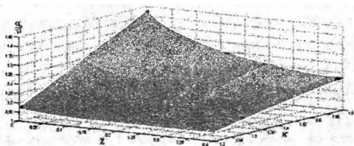
Рис. 4: Зависимость \sigma_{\text{ср}}/\sqrt{3} от \kappa и K при K_{\text{сл}} = 0,9
