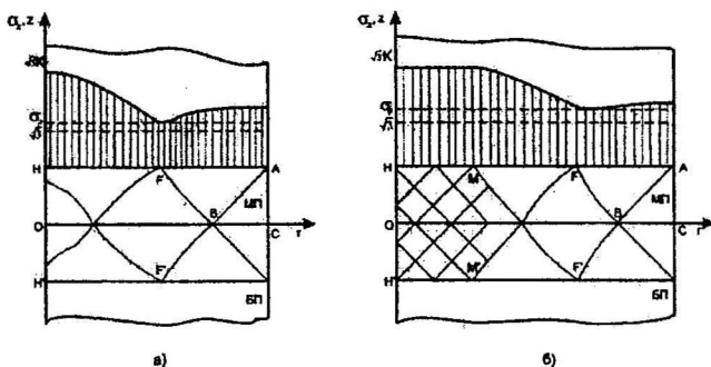
Рис. 2: Осевое сечение МП слоя и эпюра нормальных напряжений \sigma_z по контактной поверхности HA : а) первый случай – \sigma_z < \sqrt{3}K всюду на контактной поверхности; б) второй случай – существует участок HM , на котором \sigma_z = \sqrt{3}K (в области HMM'H' НС простое равномерное)
