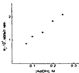
Рис. 9. Зависимость скорости реакции (2) от концентрации уксусной кислоты при 40° С и постоянном значении [AcO^-] (0.3 M).
