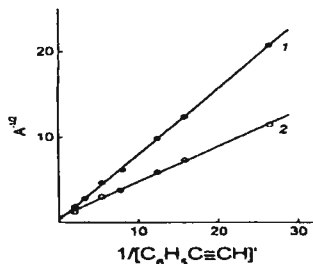
Рис. 4. Зависимость A от концентрации 50. 1. - 40°C, 2. - 50°C, [TЭА] 0.48 M , [CH_3COOH] 0.085 M .
