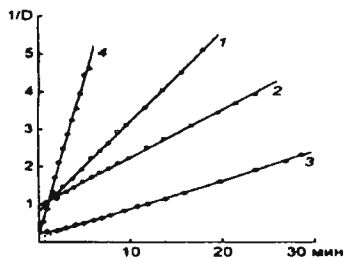
Рис.3. Примеры кинетических анаморфоз второго порядка для реакции фенилацетилена в буфере: (C_2H_5)_3N - CH_3COOH в пиридине.
