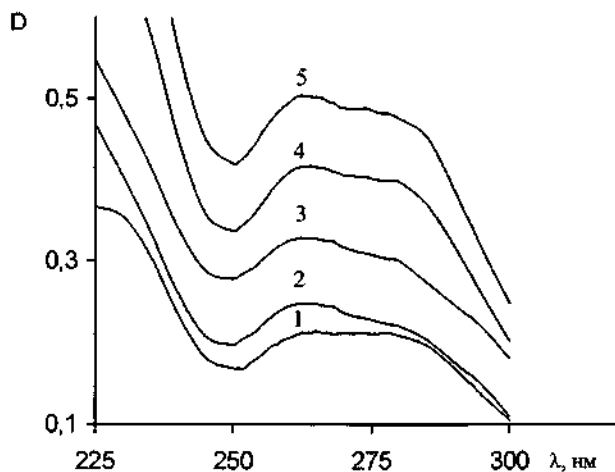
Рис. 1. Электронные спектры поглощения: 1 - элементарной серы в н - гексане; 2,3,4,5 - веществ, экстрагированных н - гексаном из осадков, полученных при фотолизе КТС.
