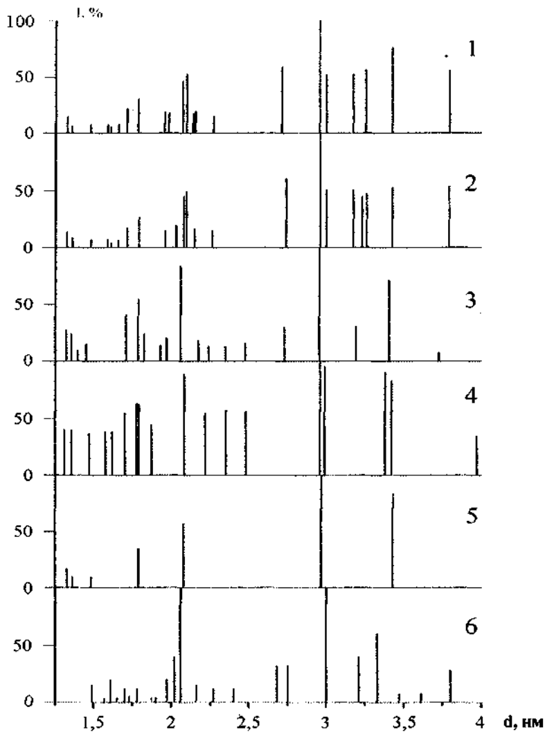
Рис. 2. Штрихрентгенограммы осадков, полученных при фотолизе КТС: 1 - в воздушной атмосфере; 2 - в инертной атмосфере; 3 - с добавкой тиомочевины в воздушной атмосфере; 4 - с добавкой тиомочевины в инертной атмосфере; 5 - сульфид свинца по литературным данным; 6 - сульфат свинца по литературным данным.
