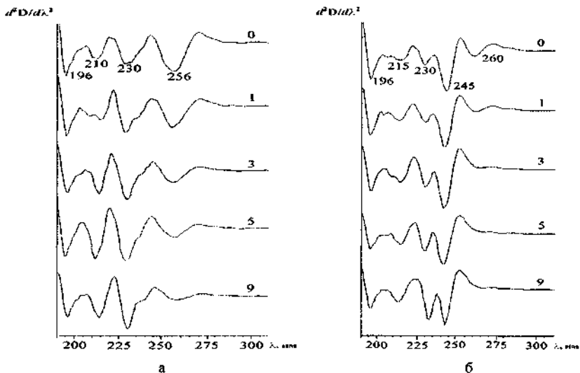
Рис. 4. Изменения в дифференцированных спектрах поглощения при фотолизе: а - водных растворов КТС ( K^{-3} M ); б - водных растворов КТС с добавкой тиомочевины ( 10^{-3} M ). Цифры у кривых соответствуют экспозициям (мин).
