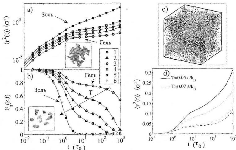
Рис. 2: а) Среднеквадратичное смещение и б) некогерентная функция рассеяния F_s(k = 7.24\sigma^{-1}, t) при различных температурах (1 – T = 0.05\epsilon/k_B ; 5 – T = 0.3\epsilon/k_B ); в) мгновенная конфигурация системы при T = 0.05\epsilon/k_B и \phi = 0.13 ; д) среднеквадратичное смещение быстрых (темные линии) и медленных (серые линии) частиц.
