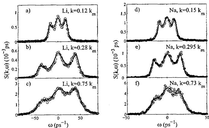
Рис. 1: Динамический структурный фактор S(k, \omega) жидкого лития [a), b), c)] при T = 475\text{K} и жидкого натрия [d), e), f)] при T = 390\text{K} : ( \circ \circ \circ ) - экспериментальные данные по неупругому рассеянию рентгеновских лучей (Scoripigno T. et al. Rev. Mod. Phys. 2005. т.77. С.881.); линия - теоретический расчет. Величина k_m - положение первого максимума в S(k) .
