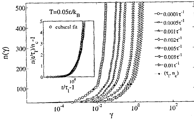
Рис. 5: Кривые роста кристаллического зародыша в стекловой системе Джугутова под внешним сдвигом при различных скоростях сдвига \dot{\gamma} и температуре T = 0.05\epsilon/k_B . Результаты соответствуют случаю неоднородной сдвиговой деформации. Вставка: Масштабированные кривые роста.
