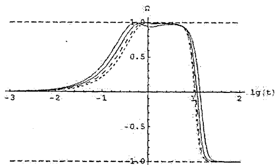
Рис.2. Эволюция космологического ускорения, в зависимости от скалярного заряда Ферми-частиц: пунктирная линия q=0 ; разреженная пунктирная линия q=0,3 ; сплошная линия q=1 ; сплошная жирная линия q=5 .
