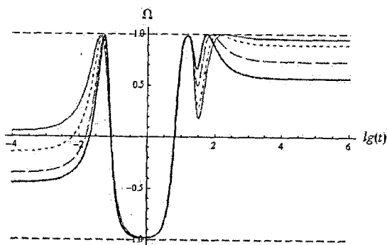
Рис.6. Эволюция коэффициента баротропы, в зависимости от массы Ферми-частиц m : пунктирная линия m=1 ; разреженная пунктирная линия m=0,95 ; сплошная линия m=1 ; сплошная жирная линия m=1,1 .
