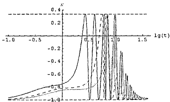
Рис.6. Эволюция коэффициента баротропы, в зависимости от массы скалярного поля: частая пунктирная линия: \mu=1 , пунктирная линия: \mu=1.2 , сплошная линия: \mu=2 .
