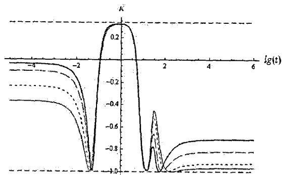
Рис.5. Эволюция коэффициента баротропы, в зависимости от массы Ферми-частиц m : пунктирная линия m=1 ; разреженная пунктирная линия m=0,95 ; сплошная линия m=1 ; сплошная жирная линия m=1,1 .
