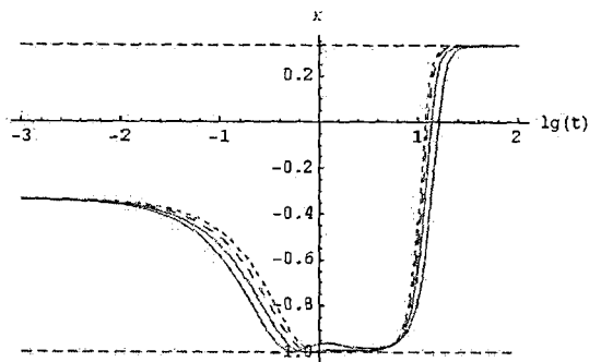
Рис.1. Эволюция коэффициента баротропы, в зависимости от скалярного заряда Ферми-частиц: пунктирная линия q=0 ; разреженная пунктирная линия q=0,3 ; сплошная линия q=1 ; сплошная жирная линия q=5 .
