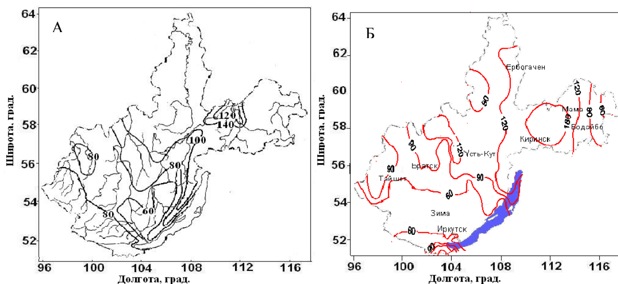
Рис. 4. Запасы воды в снежном покрове на территории Иркутской области за периоды: 1891-1960 гг. (А) и 2000-2009 гг. (Б).
