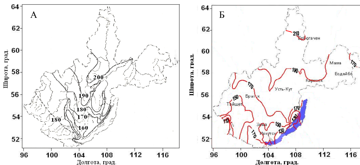
Рис. 2. Среднемноголетнее число дней со снежным покровом на территории Иркутской области за периоды: 1891-1960 гг. (А) и 2000-2009 гг. (Б).
