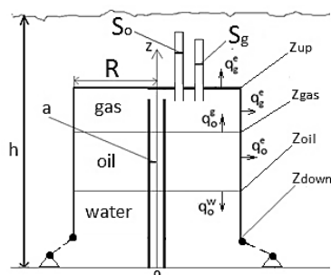
Рис. 1. Принципиальная схема "купола-сепаратора"
