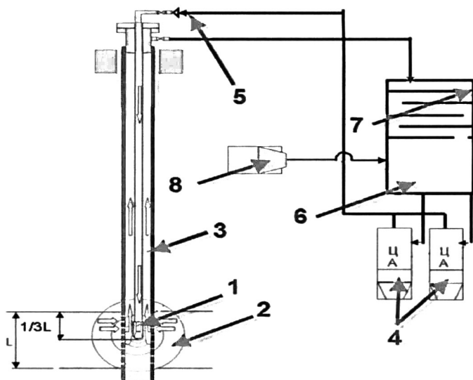
Рис. 6. Схема обвязки наземного оборудования при обработке без перемещения ГДГВ
