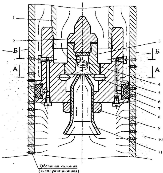
Рис. 5. Вибрационно-вакуумный очиститель зоны продуктивного пласта
