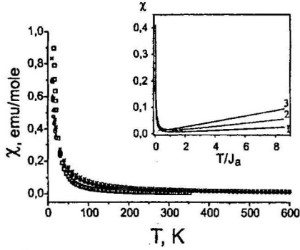
Рис. 5. Температурная зависимость восприимчивости в нулевом поле. ( \square ) – экспериментальные данные, ( \circ ) – J_f = -2321K , \delta = \frac{|J_f|}{J_a} = 2.00 ; ( \Delta ) – J_f = -696K , \delta = 1 ; \times – J_f = -23K , \delta = 0.02 – результаты модифицированной спин-волновой теории
