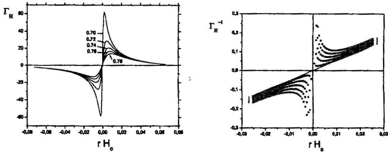
Рис. 9. (а) Магнетокалорический эффект вблизи критического поля H_c как функция контролируемого параметра \gamma . Значение энтропии на блок показано стрелкой на конце каждой линии. (б) Зависимость обратной от \Gamma_H как функции \gamma . Направление изменения энтропии от 0.70k_B до 0.78k_B с шагом 0.02k_B показано стрелками. Данные кривой S = 0.70k_B подогнаны с помощью линии 3.5785(H - H_c) - 0.0004 (пунктирная линия).
