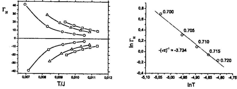
Рис. 8. Магнетокалорический эффект вблизи критического поля H_c при изменении температуры в области низких температур и при постоянном значении контролируемого параметра r : \pm 0.66 \times 10^{-3} ( \circ ), \pm 1.76 \times 10^{-3} ( \triangle ), \pm 2.76 \times 10^{-3} ( \square ) (а); "log-log" график \Gamma_H от температуры в квантовом критическом режиме r = 0 (б).
