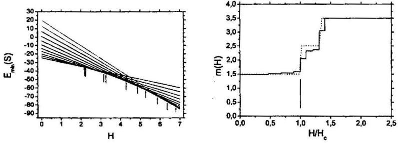
Рис. 6. (а) Схема построения кривой намагничивания при T = 0 ; (б) Кривая намагничивания ферромагнитной цепочки (5/2, 1) при T = 0 , восстановленная по спектру системы из N = 9 узлов. Скачок намагниченности при критическом поле H_c = 3.04 J отмечен стрелкой. Результат DPIR расчета для низких температур ( T = 0.001 J ) показан для сравнения.
