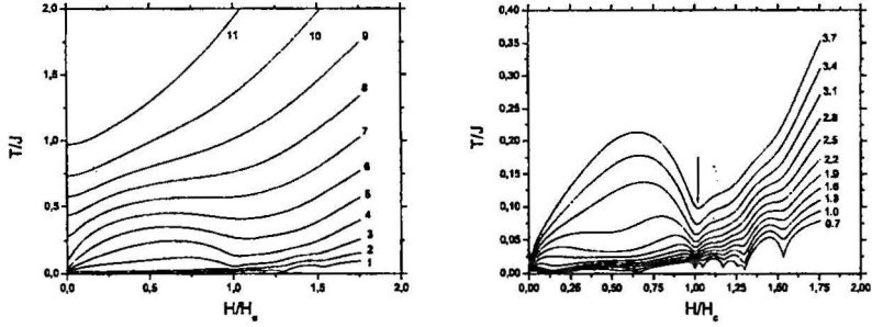
Рис. 7. Кривые постоянной энтропии для ферромагнитной цепочки (5/2,1) в большом (а) и малом (б) масштабах. Значения энтропии на блок S/N , измеренные в единицах k_B , отмечены числами на конце каждой линии. Наклон вблизи предполагаемой квантовой критической точки показан стрелкой.
