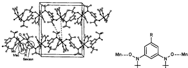
Рис. 1. Пространственный вид (а) и схема цепочечной структуры соединения [Mn(hfac)_2BNO_R] (б).
