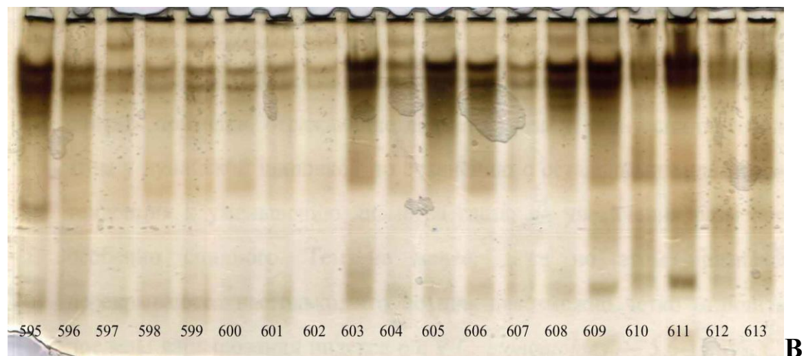
Рис. 4.1. Изменчивость и полокусная интерпретация спектров неспецифических эстераз у особей Lymnaea stagnalis s. lato разных популяций: А – №№ 5-14 р. Тетерев, окрестности г. Житомира, №№ 15-20 – р. Псел (фиксация альтернативных аллелей по локусу Es-4 ); Б – Нижний Днепр, г. Голая Пристань (полиморфизм локуса Es-4 ); В – р. Тетерев, окрестности г. Коростень (фиксация генотипа Es-4 aa ).
