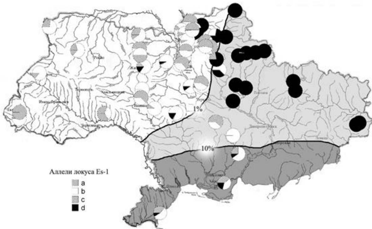
Рис. 6.5. Изменчивость частот аллелей локуса Es-1 в популяциях катушки роговидной P. cornutus в пределах Украины, на фоне изолиний, показывающих распределение относительного числа засушливых дней в году
