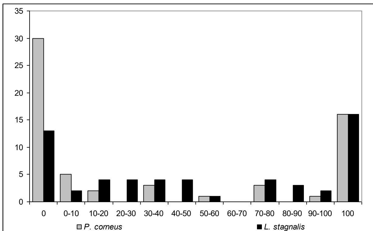
Рис. 6.2. Распределение частот аллелей локусов неспецифических эстераз, диагностирующих восточные алловиды двух надвидовых комплексов легочных моллюсков
