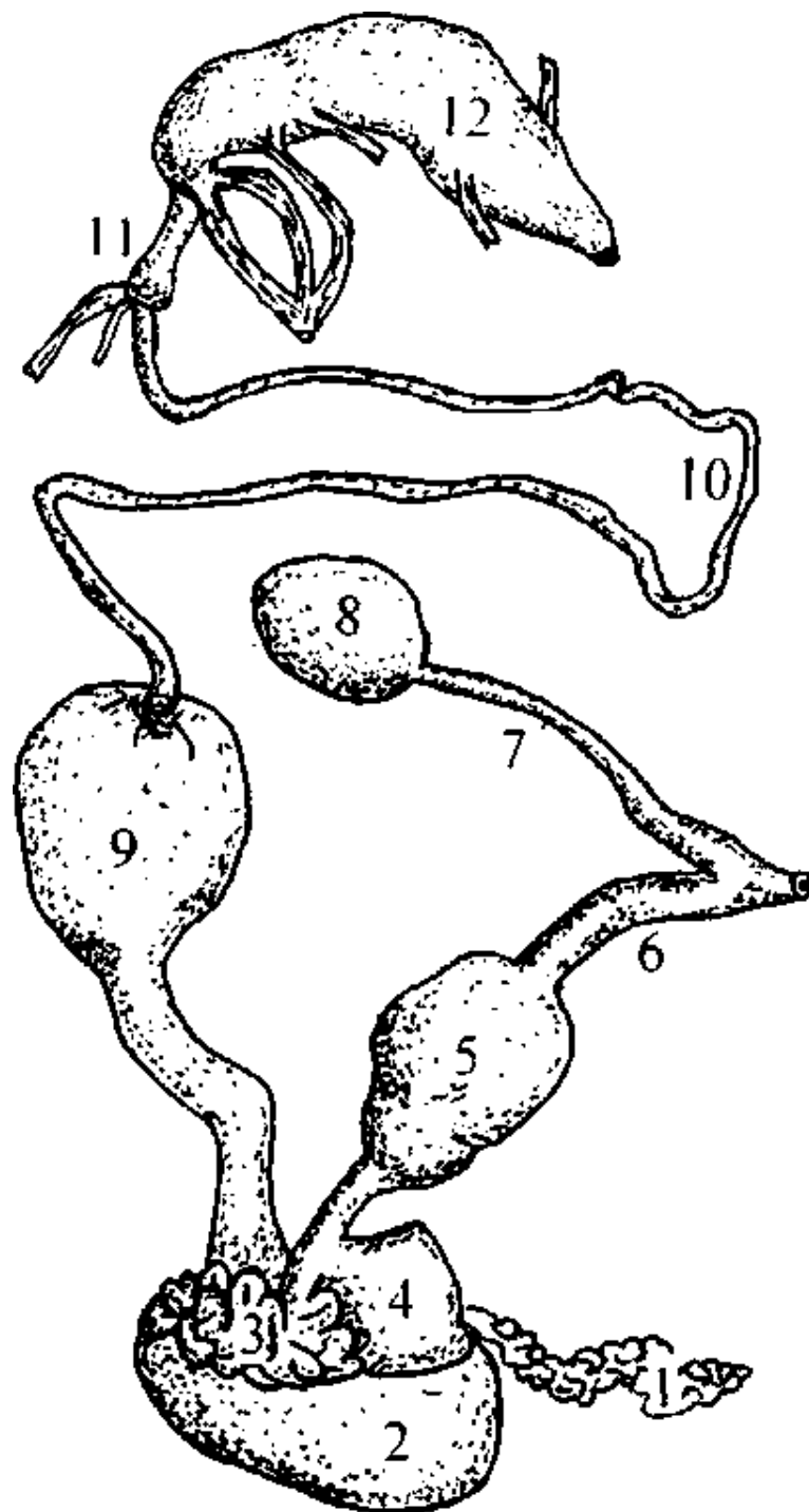
Рис. 2.3. Половая система Lymnaea stagnalis (Linnaeus, 1758) по М. Яцкевич (Jackiewicz, 1998):
