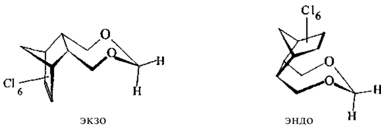
Рис.2. Конформеры ГХА
