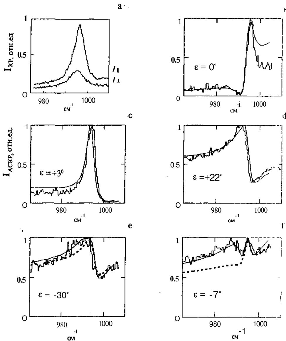
Рис.1. КР спектры (a) и АП АСКР спектры (b - f) жидкого ХЦГ (T = 293 K). Ступенчатая линия - экспериментальные спектры, сплошной линией показаны рассчитанные спектры (параметры приведены в табл.1); пунктирная линия в (e) и (f) - спектры, рассчитанные без полосы 992 см -1 .
