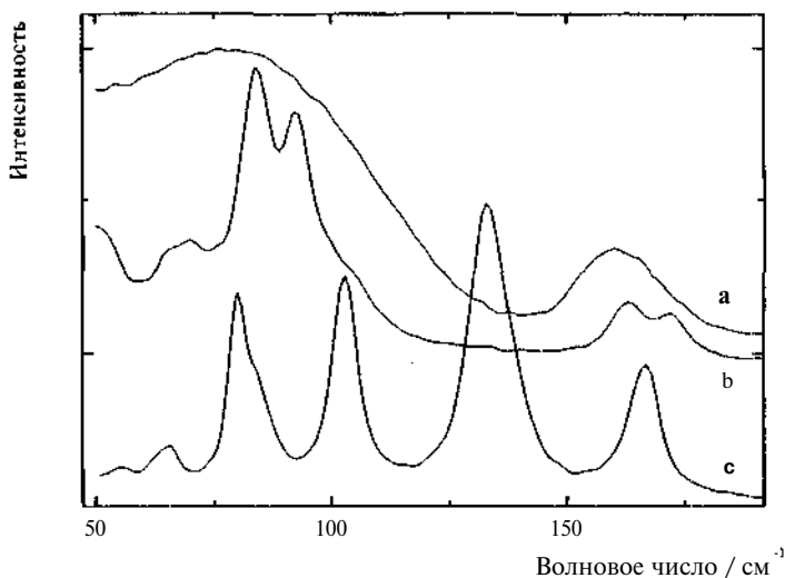
Рис. 4. Спектры КР ЭБ: а - жидкость при 170K, б - кристалл А (120K) и с - кристалл В (160K).
