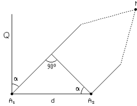
Рис. 1. Фазовый метод определения угла направления на метеорный след; A_1 , A_2 – антенны фазового угломера; d – база угломера; M – зеркальная точка на метеорном следе; \alpha – угол цели; Q – плоскость, нормальная к базе угломера
