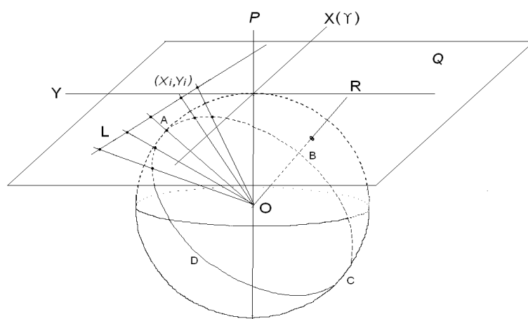
Рис. 5. Графическая иллюстрация применения метода Джонса – Мортон при определении экваториальных координат радианта метеорного потока
