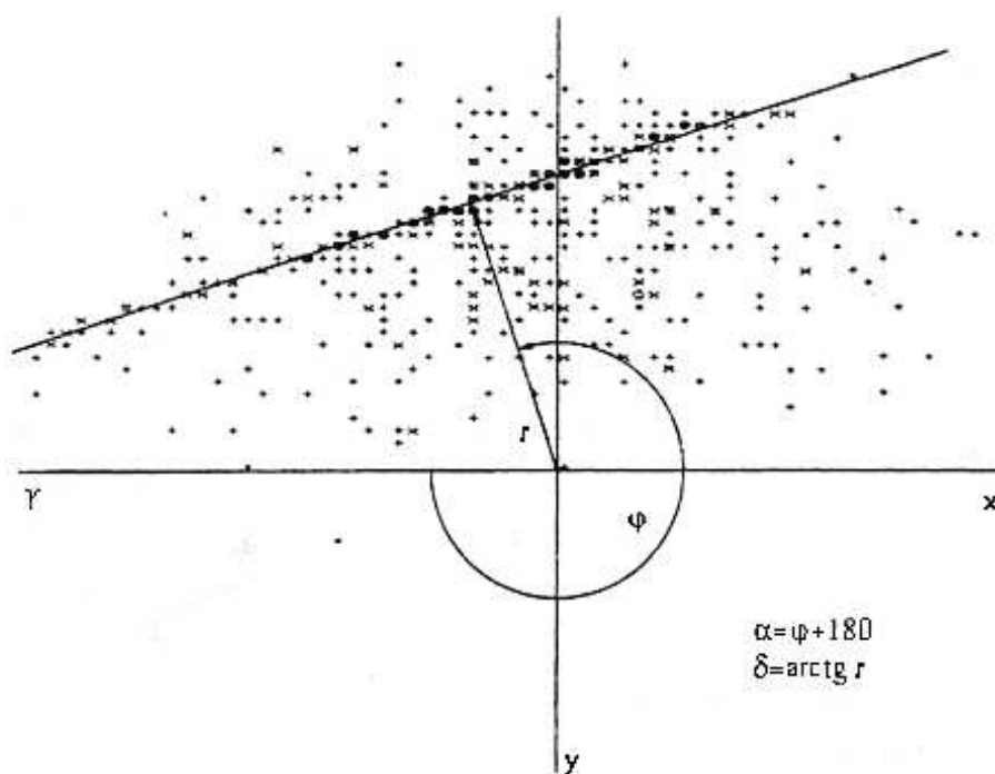
Рис. 6. Проекция зеркальных точек, зарегистрированных в период действия потока Геминид, на плоскость ( Q ): + – одиночная точка; \times , * , \bullet – наложение 2, 3, 4 и более точек; \gamma – точка весеннего равноденствия; \alpha – прямое восхождение и \delta – склонение радианта метеорного потока
