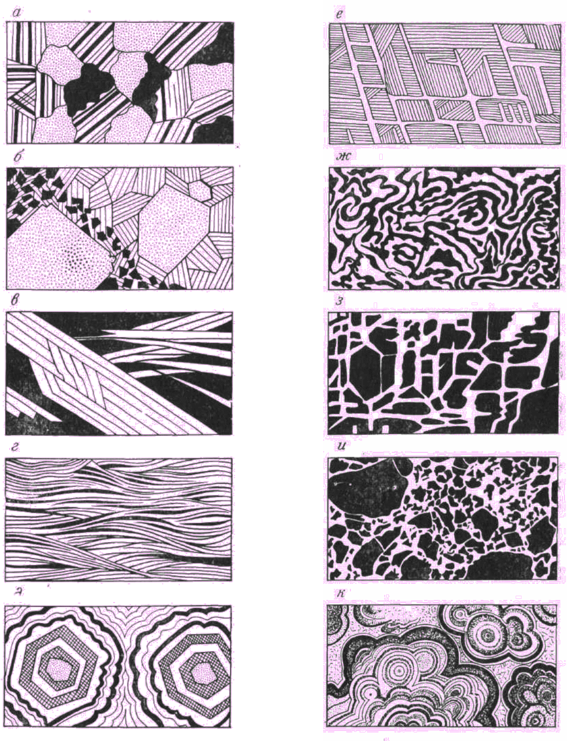
Рис. 6. Некоторые типы структур руд (схемы).
