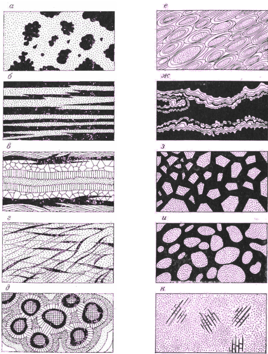
Рис. 1. Некоторые типы текстур руд (схемы).
