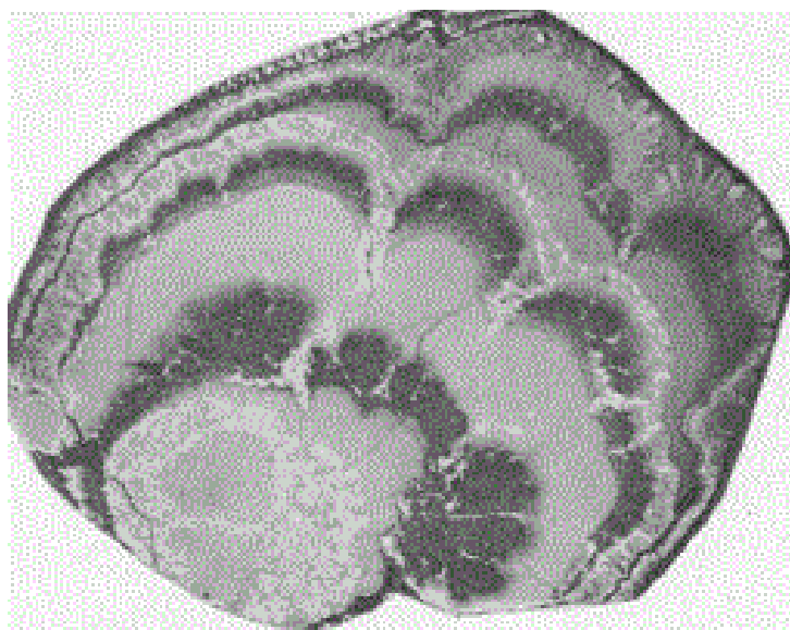
Рис. 5. Колломорфная текстура агрегата псиломелана (светло-серое), с трещинками усыхания и халцедона (черное). Структура агрегата псиломелана и халцедона гелевая. Для пиролюзита (белое) характерны волокнистая метакolloидная структура и колломорфная метакolloидная текстура. Полированный штуф.
