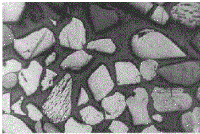
Рис. 8. Обломочная структура агрегата рутила, ильменита (белое), циркона (серое, рельефное) и кварца (черное). Обломки минералов сцементированы дикситом (черное). Полированный шлиф.
