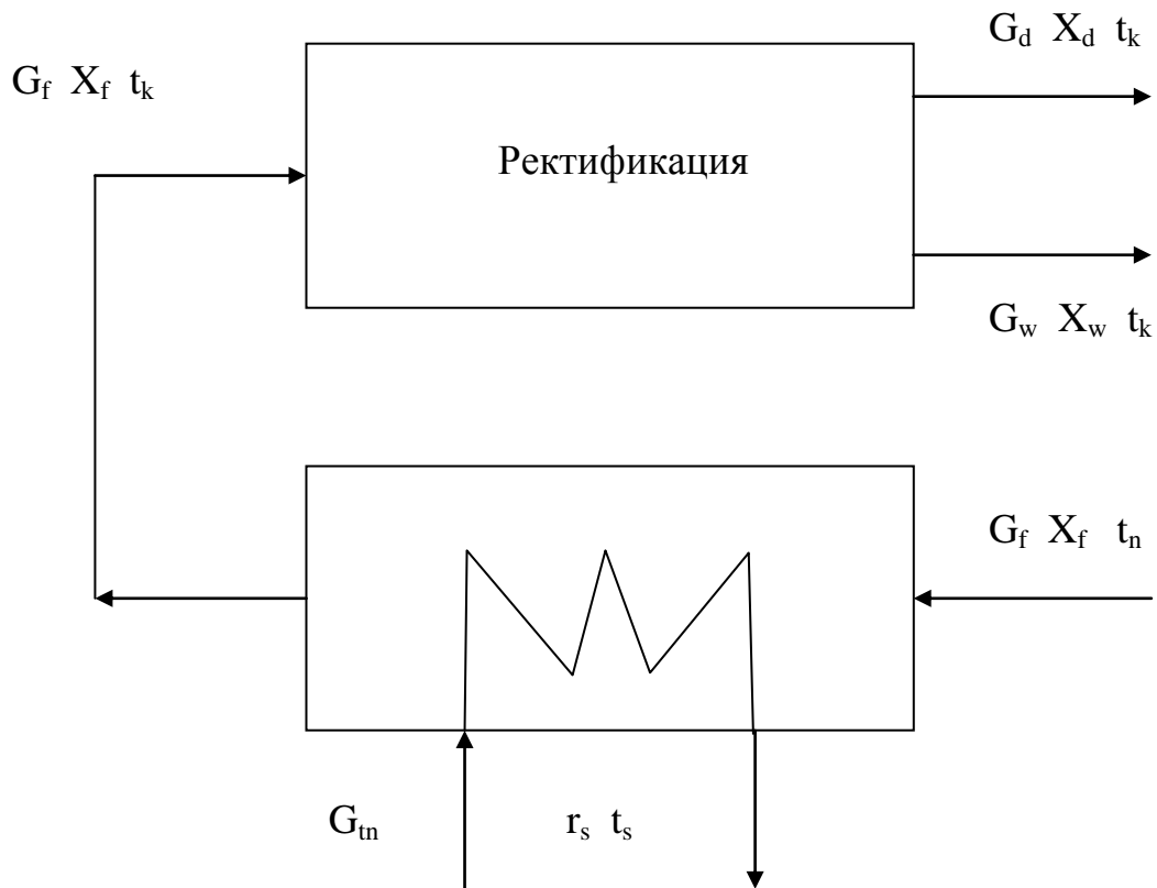
Рис. 1. Пример оформления структурной схемы
