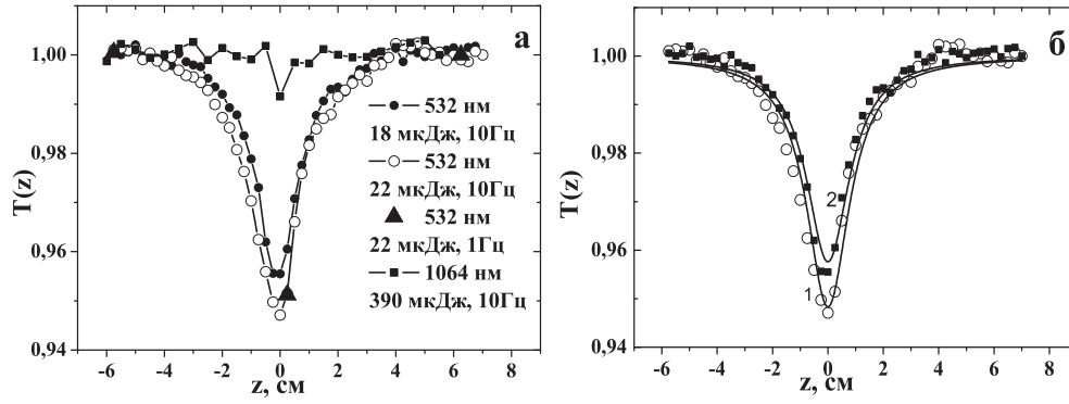
Рис. 3. а) Зависимости нормированного пропускания T(z) образца \text{SiO}_2:\text{Cu} от его положения относительно фокуса линзы ( z = 0 ) при измерении по схеме без диафрагмы; б) аппроксимация зависимости T(z) при E = 22 \mu\text{Дж} (1) и E = 18 \mu\text{Дж} (2) функцией (2)
