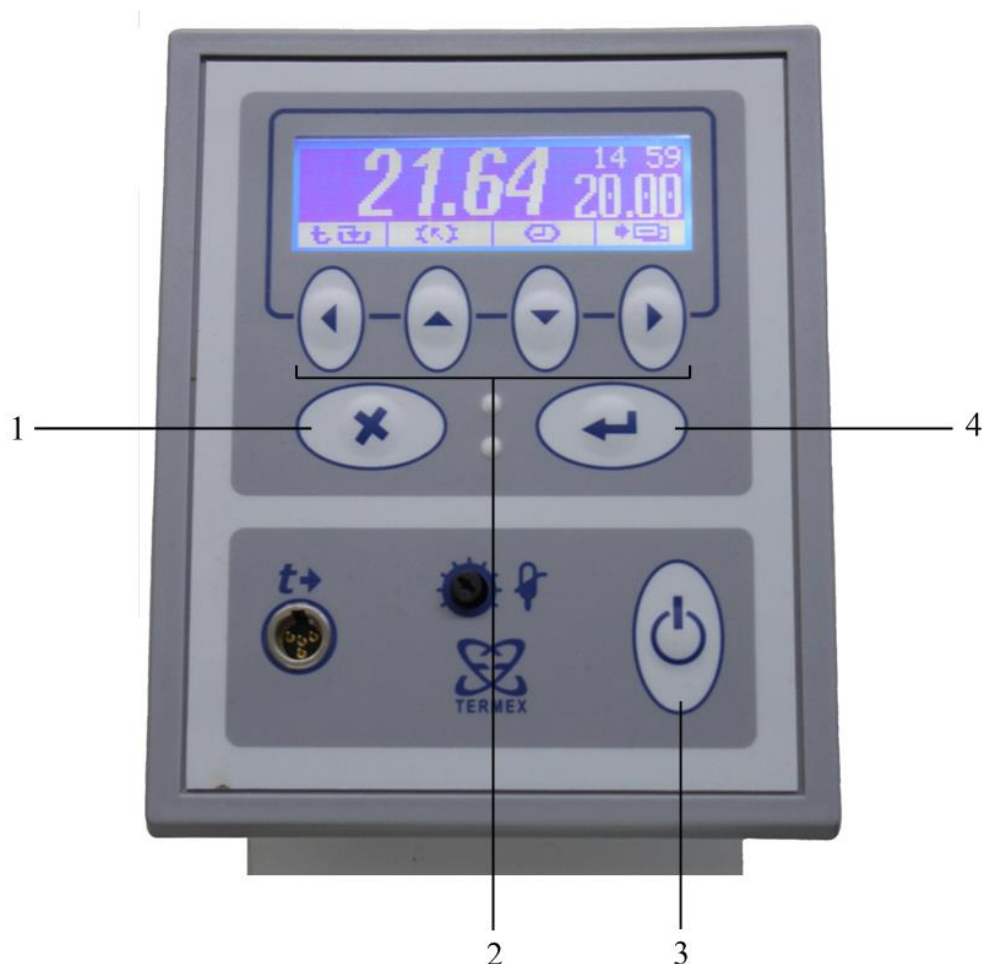
Рис. 1.6. Передняя панель блока регулирования температуры жидкостного термостата модельного ряда ВТ. Позиции: 1 – отмена действия; 2 – установка параметров и управление режимами; 3 – включение / выключение блока; 4 – подтверждение действия
