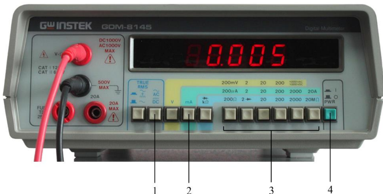
Рис. 3.3. Передняя панель мультиметра GDM-8145. Позиции: 1 – выбор режима измерения постоянного (DC) или переменного (AC) тока / напряжения; 2 – режим измерения силы тока; 3 – пределы измерений; 4 – включение / выключение прибора
