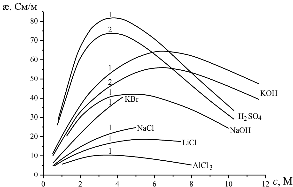
Рис. 1.1. Влияние концентрации некоторых электролитов на удельную электропроводность их водных растворов при температурах 25 (1) и 18 °C (2)
