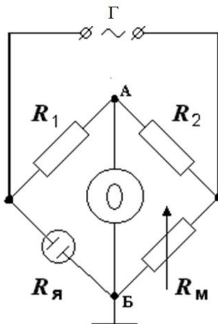
Рис. 1.4. Схема моста переменного тока для определения сопротивления раствора. R_1 , R_2 – сопротивления, R_{\text{я}} – сопротивление ячейки с раствором, R_{\text{м}} – магазин сопротивлений, \Gamma – генератор переменного тока, 0 – осциллограф
