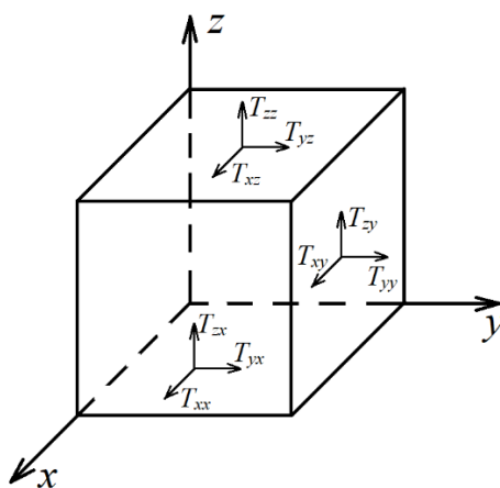
Рис.4. Пример направленности напряжений на гранях твердого тела
