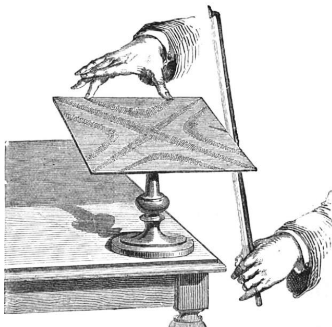
Рис.1. Способ получения фигур Хладни
