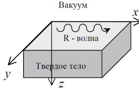
Рис.8. Образование поверхностной волны Рэлея на границе твердого тела с вакуумом
