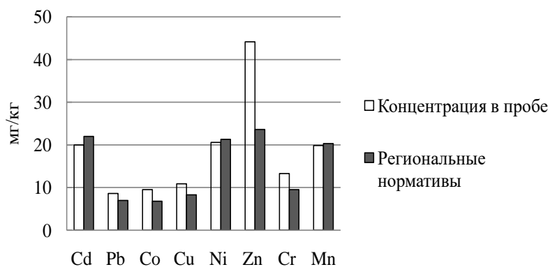
Рисунок 1 – Содержание ТМ в почвах водосборной территории Cd \times 10^2 ; Mn \times 10^{-2}
