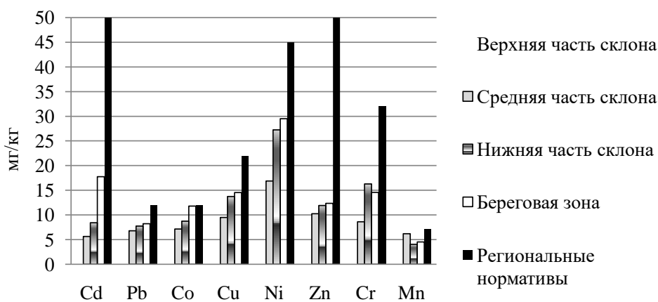
Рисунок 1 – Содержание ТМ в почвах водосборной территории Cd \times 10^2 ; Mn \times 10^{-2}
