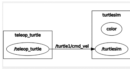
Рис. 4.10: Схема взаимодействия между нодами.
