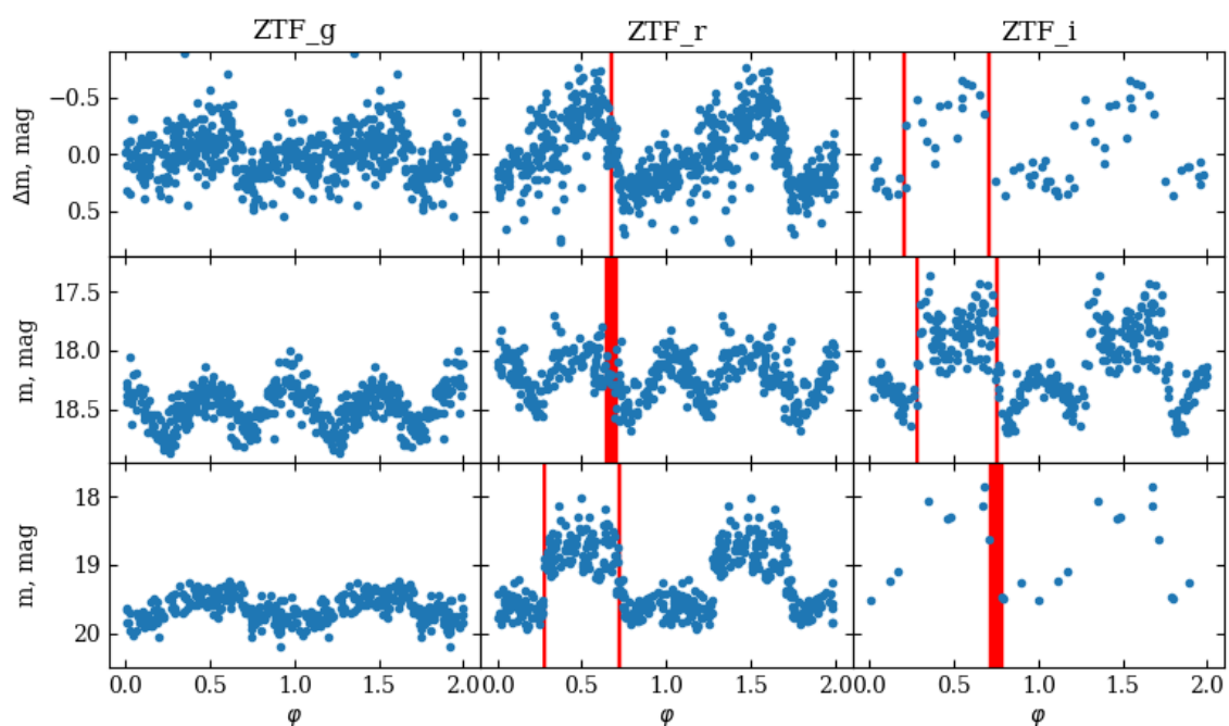
Рис. 2. Фазовые кривые блеска ВМ СгВ по данным обзора ZTF. Сверху вниз перечислены состояния блеска поляр: высокое, промежуточное, низкое. Слева направо перечислены фотометрические фильтры ( g , r , i ). Данные, использованные для построения этих кривых блеска, указаны на рис. 1. Блеск поляр в высоком состоянии отсчитывается относительно аппроксимирующих полиномов, показанных на рис. 1. Вертикальные полосы указывают моменты входа в яркую фазу и выхода из нее, ширины полос соответствуют ошибкам определения границ яркой фазы.
