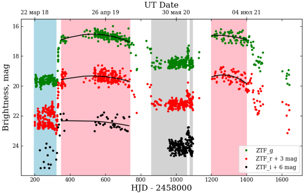
Рис. 1. Кривые блеска ВМ СгВ по данным обзора ZTF в полосах g , r , i . Области, закрашенные розовым, серым и голубым цветами указывают на высокое, промежуточное и низкое состояния ВМ СгВ соответственно. Данные, попадающие в эти области, использовались для анализа кривых блеска в трех состояниях. Черные линии — полиномы второй степени, аппроксимирующие кривые блеска в высоком состоянии.
