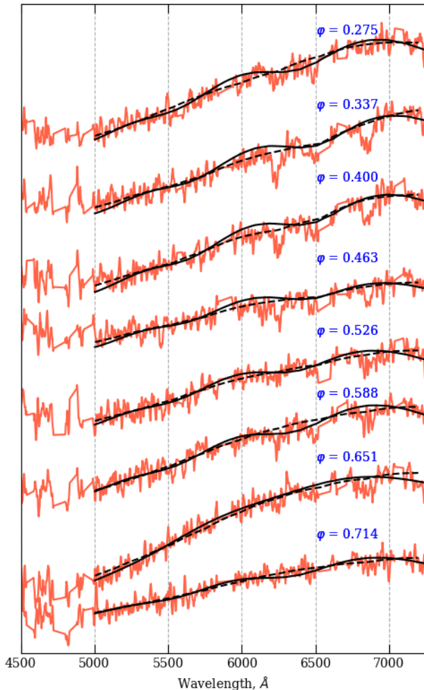
Рис. 8. Циклотронные спектры ВМ CrB (розовые линии), и их описание модельными спектрами аккреционных пятен с температурами T_e = 10 кэВ (пунктирная черная линия) и T_e = 20 кэВ (непрерывная черная линия). Указаны фазы середин экспозиции наблюдаемых спектров, найденные по эфемеридам (1).
