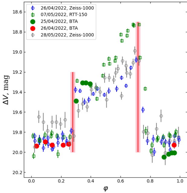
Рис. 3. Кривые блеска ВМ СгВ, полученные нами на телескопах Цейсс-1000, РТТ-150 и БТА. Вертикальными линиями указаны моменты входа в яркую фазу и выхода из нее.
