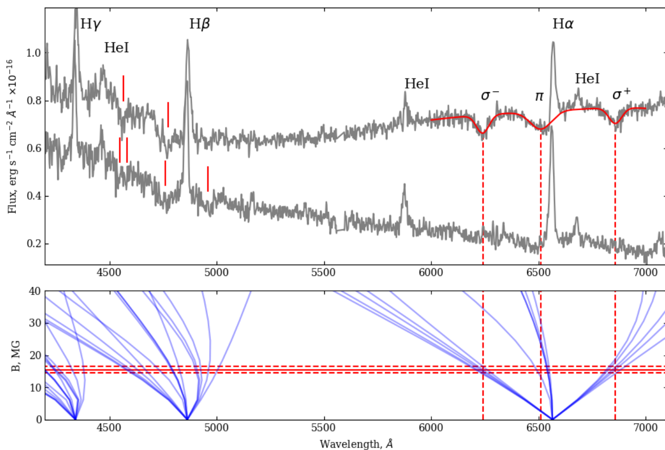
Рис. 4. На верхней панели показаны усредненные спектры VM Sgr, полученные в яркой фазе и фазе плато. Красной линией показана аппроксимация участка спектра с зеемановскими компонентами линии H\alpha комбинацией полинома и гауссиан. Вертикальными пунктирными линиями указано положение зеемановских компонент. Вертикальными непрерывными линиями указаны компоненты расщепления линии H\beta . На нижней панели представлена диаграмма положения компонент зеемановского расщепления линий H\alpha , H\beta и H\gamma для диапазона напряженности магнитного поля 0 – 40 МГс. На диаграмме горизонтальными линиями указано найденное значение магнитного поля B = 15.5 \pm 1 МГс.
