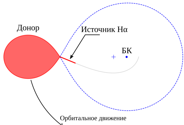
Рис. 7. Модель полюра, полученная из анализа кривых лучевых скоростей и потоков основной компоненты линии H\alpha . На рисунке указаны: звезда-донор, заполняющая свою полость Роша, белый карлик (БК), полость Роша белого карлика (пунктирная линия), баллистическая траектория частицы, испускаемой из точки Лагранжа L_1 (серая линия), источник основной компоненты линии H\alpha .
