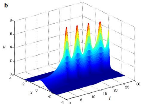
Рис. 3. Эволюция гауссова импульса огибающей в нестационарной среде при \alpha, f' = 0 : а) \beta = 0.5, \gamma = -1 + 0.01 \sin 2\pi t ; б) \gamma = -1, \beta(t) = -0.5 for t \leq 5 and \beta(t) = 0.5(1 + 0.2 \sin 2\pi t) for t > 5 ; случаи отрицательной нелинейности
