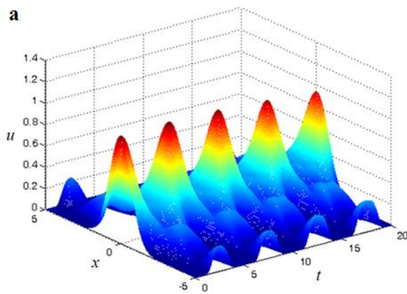
Рис. 3. Эволюция гауссова импульса огибающей в нестационарной среде при \alpha, f' = 0 : а) \beta = 0.5, \gamma = -1 + 0.01 \sin 2\pi t ; б) \gamma = -1, \beta(t) = -0.5 for t \leq 5 and \beta(t) = 0.5(1 + 0.2 \sin 2\pi t) for t > 5 ; случаи отрицательной нелинейности
