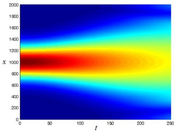
Рис. 1. Эволюция гауссовского импульса огибающей (а) при A = 2, l = 2; \beta = 0.5, \gamma = 0
