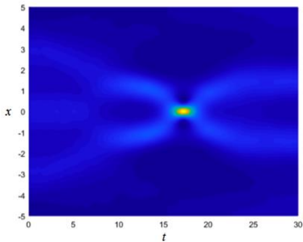
Рис. 4. Взаимодействие трех импульсов GNLS (стационарная среда) при \gamma = -1 , \beta = 0.25 ; случай слабой отрицательной нелинейности
