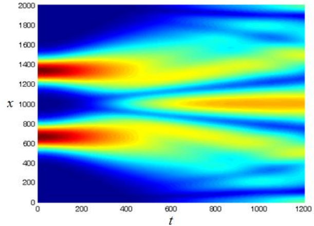
Рис. 2. Эволюция гауссовского импульса огибающей (б) при A = 1, l = 4; \beta = 0.5, \gamma = 0
