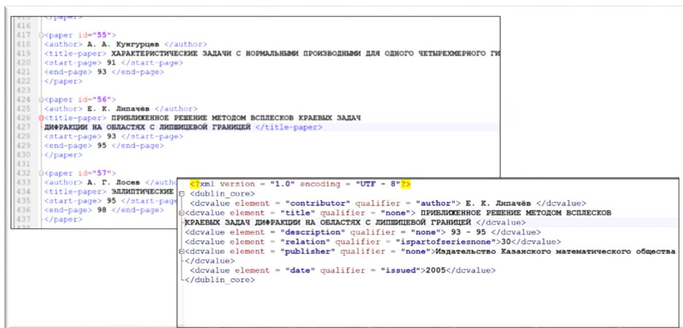
Рис. 1. Преобразование метаданных в спецификацию Dublin Core с учётом специфики цифрового хранилища DSpace.
