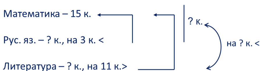
Рис. 3. Краткая запись ко второй задаче
