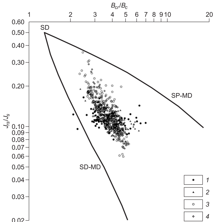
Рис. 4. Характеристики магнитной структуры зерен по гистерезисным параметрам осадков оз. Большое Яровое на теоретической диаграмме Дзю—Данлопа.
