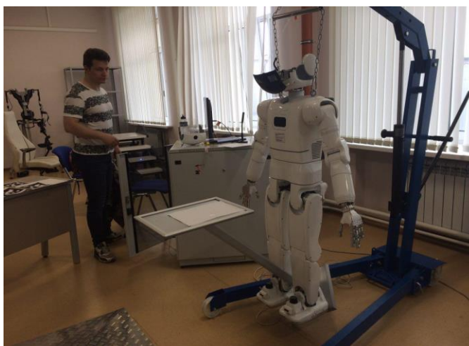
Рисунок 2. Подготовка оборудования и робота AR-601M к экспериментам. На фото – соавтор А.Г.Сагитов.
