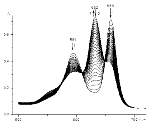
Изменение ЭСП H_2Pa(C_6H_4CF_3)_8 в присутствии морфолина в течение 30 мин при 323 К и C_{Mor} = 10.90 (моль/л) в системе бензол – 5% ДМСО
