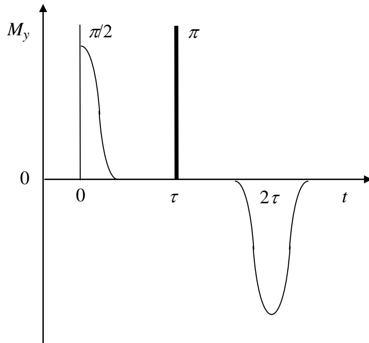
Fig. 6. Spin echo.
