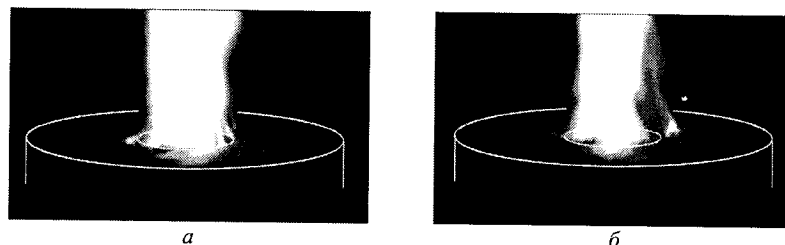
Рис. 5. Мгновенные фотографии прикатодной области плазменного столба. Белыми линиями обозначены очертания пористой пластины. Экспозиция 67 мкс. Интервал между кадрами 125 мс, d = 23 мм, \langle I \rangle = 6 А
