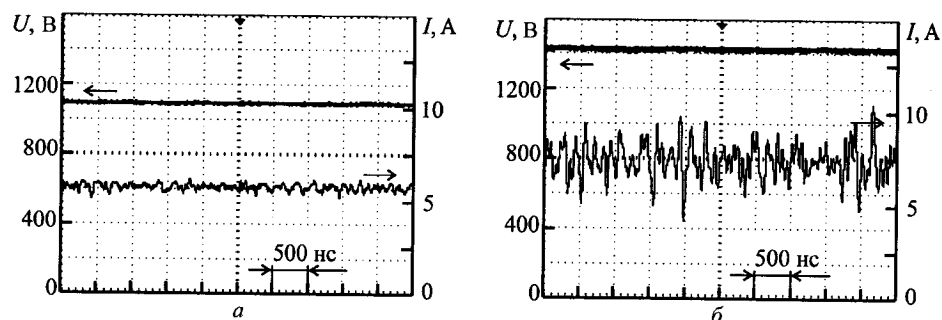
Рис. 4. Осциллограммы токов и напряжений. l = 10 см: а – электролит истекает из цилиндрического канала с диаметром D = 75 мм; б – на выходе канала установлена пористая пластина с отверстием d = 23 мм
