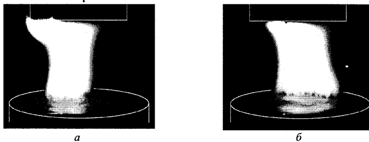
Рис. 3. Фотографии газового разряда. Экспозиция 196 мкс. Белыми линиями обозначены внешние очертания анода и стенки канала, из которого истекает электролит. D = 75 мм, l = 5 см, I = 4 А, U = 840 В
