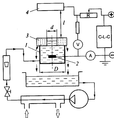
Рис. 1. Принципиальная схема экспериментальной установки. Стрелками указано направление движения электролита
