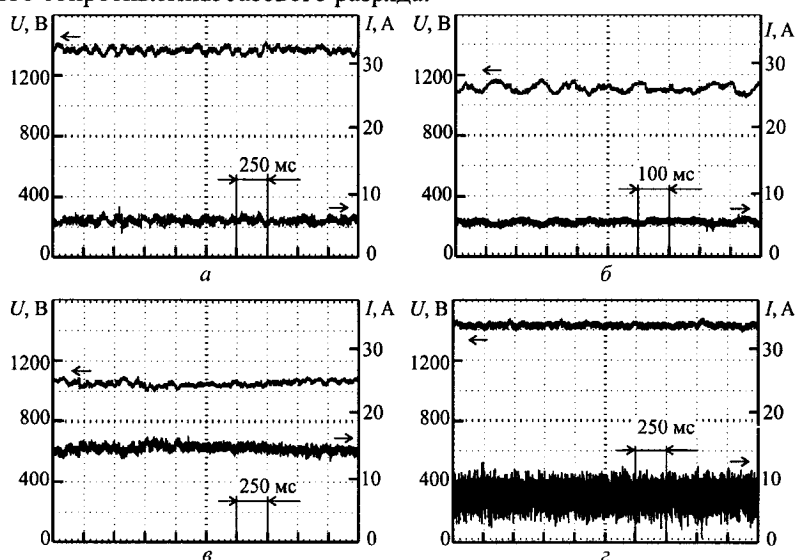
Рис. 2. Осциллограммы токов и напряжений: а – D = 20 мм, l = 10 см; б – D = 75 , l = 10 ; в – D = 75 , l = 5 ; з – d = 23 мм, l = 10 см
