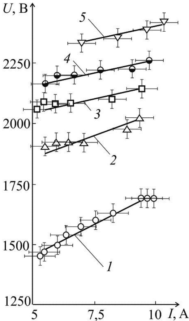
Рис. 5. Вольтамперные характеристики (вариант В). Диаметр отверстия в пористой пластине d = 21 мм. Межэлектродное расстояние l : 1–15 см; 2–25 см; 3–30 см; 4–35 см; 5–40 см.
