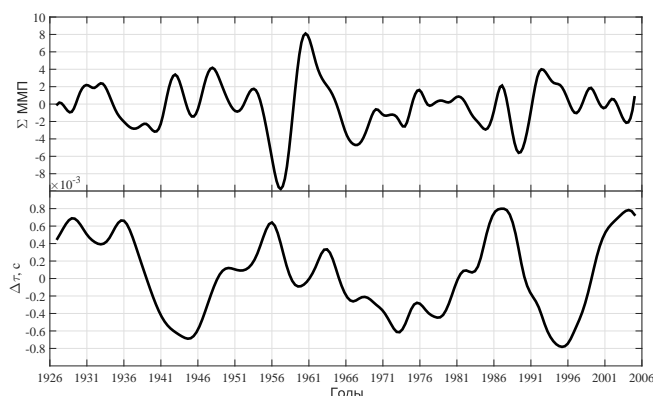
Рис. 3. Месячные суммы ежедневных полярностей секторов ММП ( \Sigma ММП) и колебания продолжительности суток ( \Delta\tau ) за 1926–2006 гг.
