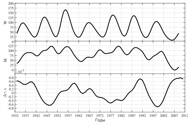
Рис. 1. Числа Вольфа ( W ), индексы магнитной возмущенности ( M ) и колебания продолжительности суток ( \Delta\tau ) за 1933–2009 гг. (17–24 циклы по цюрихской нумерации)
