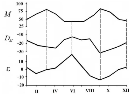
Рис. 4. Средние циклические кривые индекса магнитной возмущенности ( M ), D_{st} – вариаций и угловых ускорений вращения Земли ( \varepsilon )
