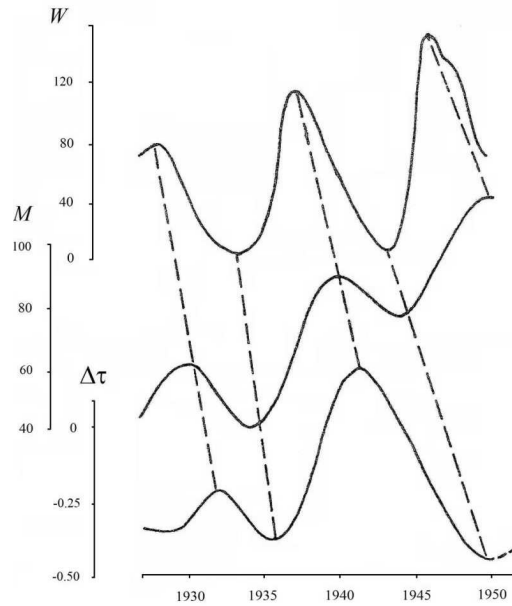
Рис. 2. Числа Вольфа ( W ), индексы магнитной возмущенности ( M ) и колебания продолжительности суток ( \Delta\tau ), построенные по реперным фазам W и M за 1927–1950 гг.
