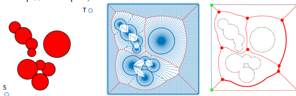
Рисунок 5. Среда с препятствиями (слева), процедура построения графа Вороного (посередине), путь на графе Вороного (справа).
