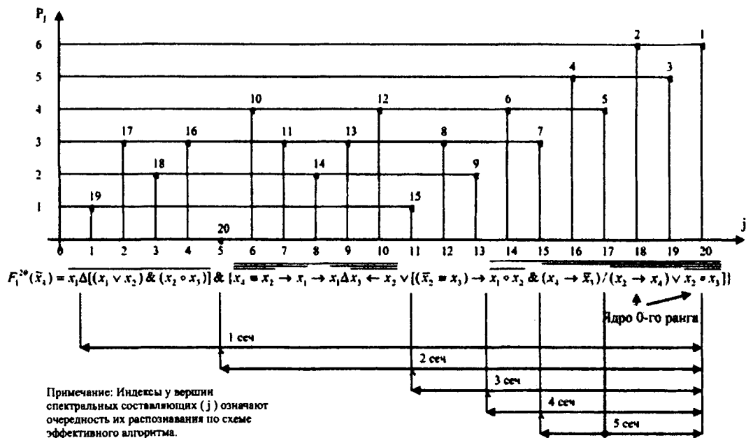
Рис. 2. Выбор 1-го шага для получения эффективного алгоритма A: F_{\eta}^{\ell}(\tilde{x}_n) \Rightarrow f_k(\tilde{x}_n)
