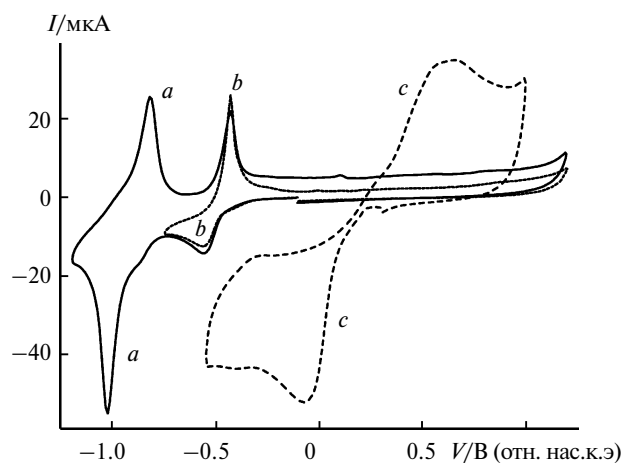
Рис. 1. ЦВА-кривые р(MVCA 8+ -co-St) (1 мг · мл -1 , ~2.0 мМ MV 2+ ) ( a, b ) и 2 \cdot 10^{-3} М [PdCl 4 ] 2- ( c ); E_r = -1.20 ( a ), -0.75 ( b ), -0.55 В ( c ).
